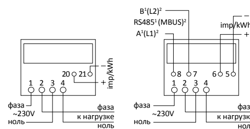
Схема включения счетчика НЕВА 101, НЕВА 104
